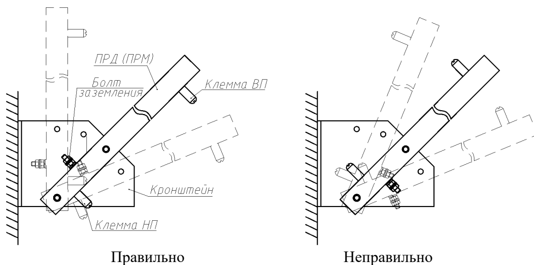
Рисунок 2.6 – Установка ПРД и ПРМ
